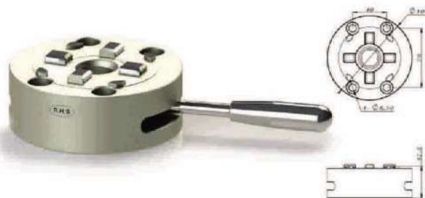
D100 3M Manual Chuck
